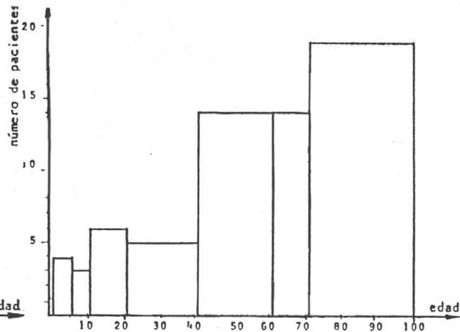
HISTOGRAMA INCORRECTO
