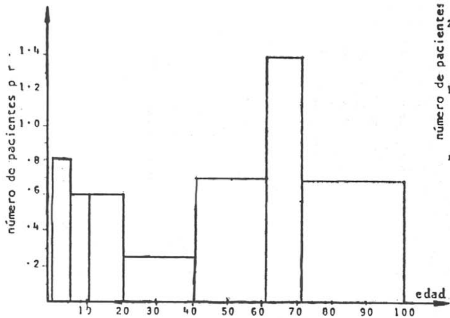
HISTOGRAMA CORRECTO
